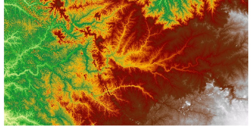
Un ejemplo de mapa de elevación de África central con una resolución espacial de 90 m (Tile 42_12).
