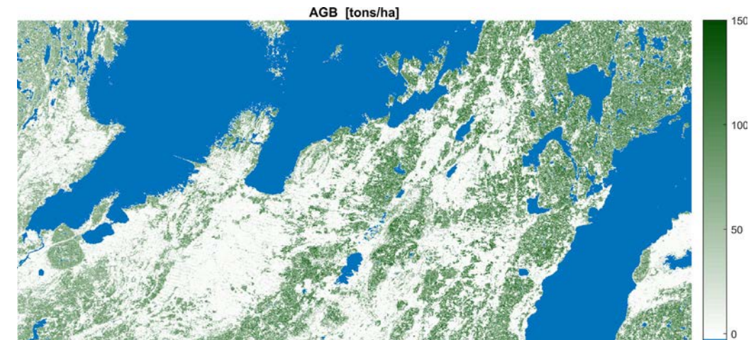
Biomasa forestal medida por Sentinel-1 de Copérnico. Fuente de la Imagen: ESA
