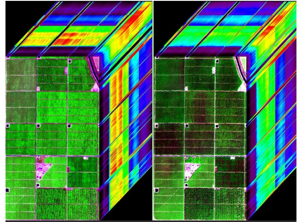
Imágenes de AVIRIS de mayo (izq.) y noviembre (der.) 2011 del estrés hídrico de huertos en California para evaluar el NDMI. Fuente de la Imagen: Hunt et al
