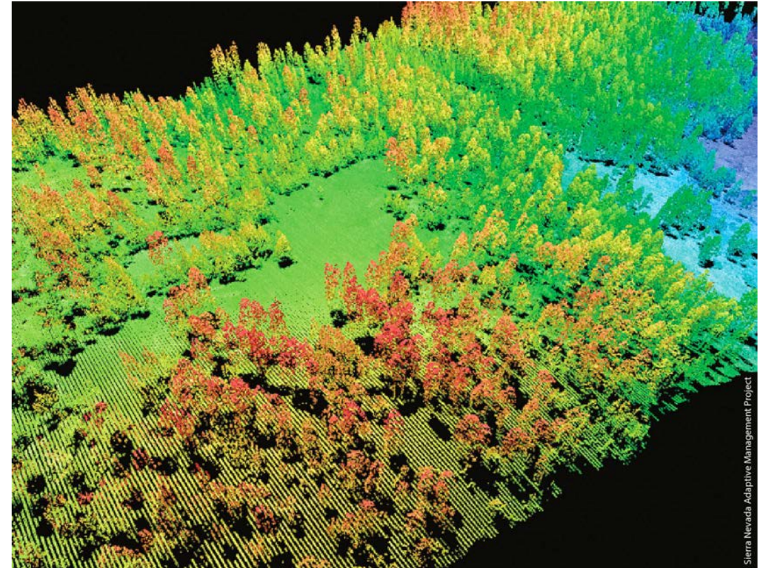
Puntos Lidar muestran árboles en el Bosque Nacional Sierra donde se ha realizado gran parte de la investigación sobre la teledetección. Fuente de la Imagen: Keley y Tommaso, 2015
