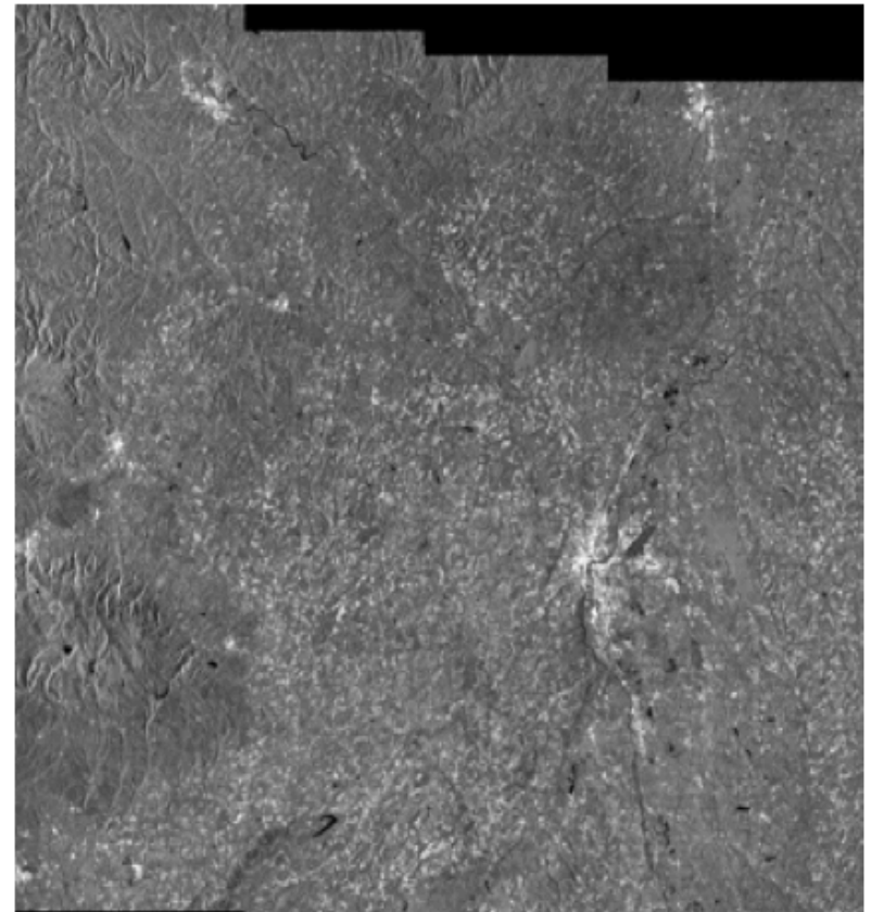
TSX-TOPS image
